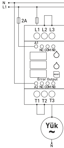
Bağlantı Şeması (Monofaz)
