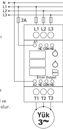
Bağlantı Şeması (Trifaz)
